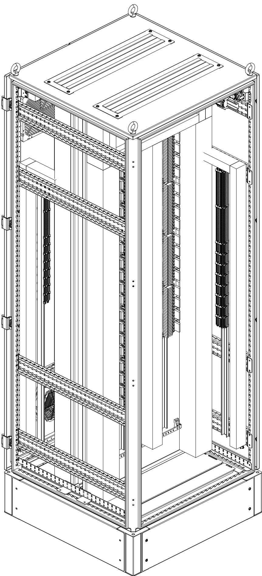
СВ изометрия
