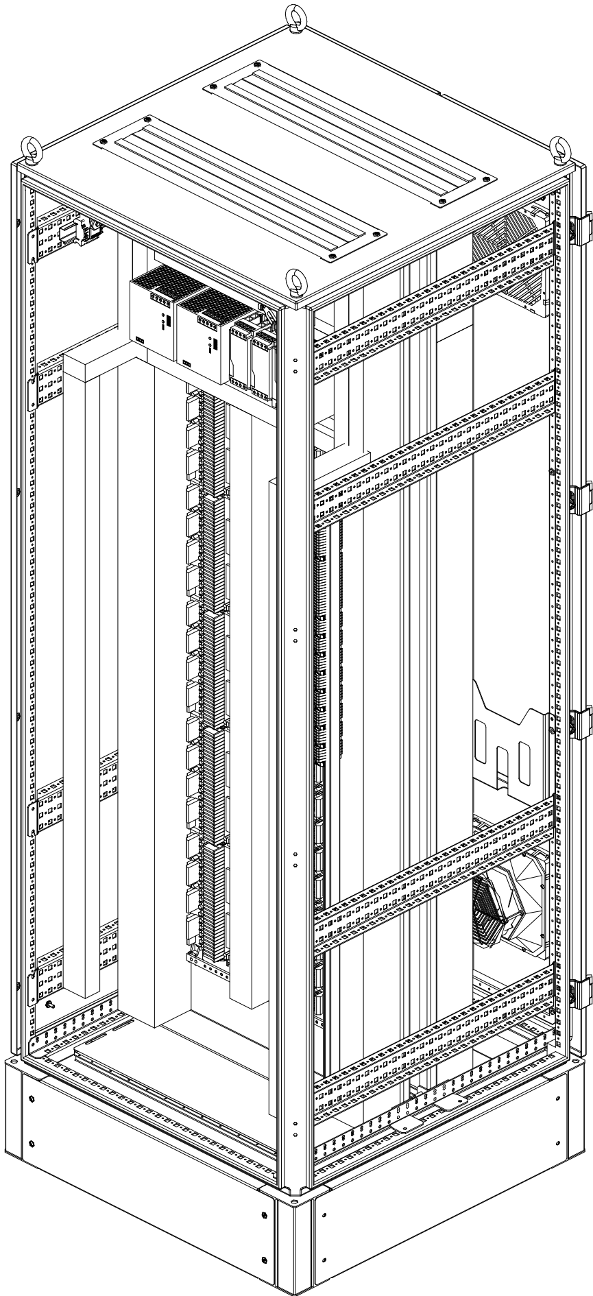
ЮВ изометрия
